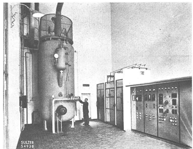
Hochspannungs-Elektrodampfkessel von 4000 kW, 12000 Volt, 13 atü in einer chemischen Fabrik, mit Hoch- und Niederspannungs-Schaltanlage.
