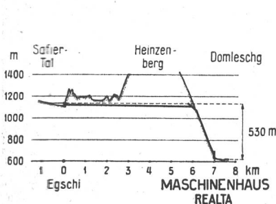
Abb. 2 Längenprofil.
