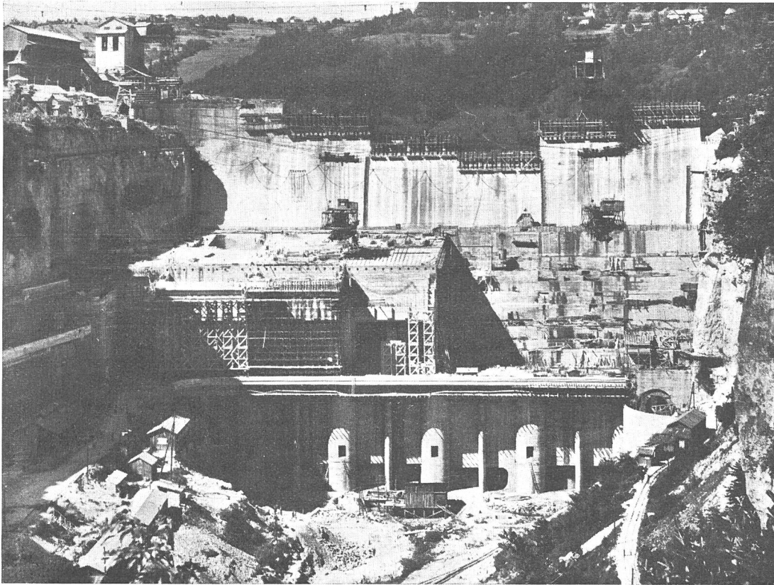
Usine de Génissiat sur le Rhône en construction
