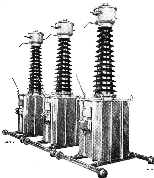
Meßgruppe 150 kV
