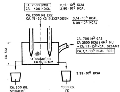
Abb. 3 Elektro-Niederschachtofen, schematische Darstellung mit Anhaltszahlen
