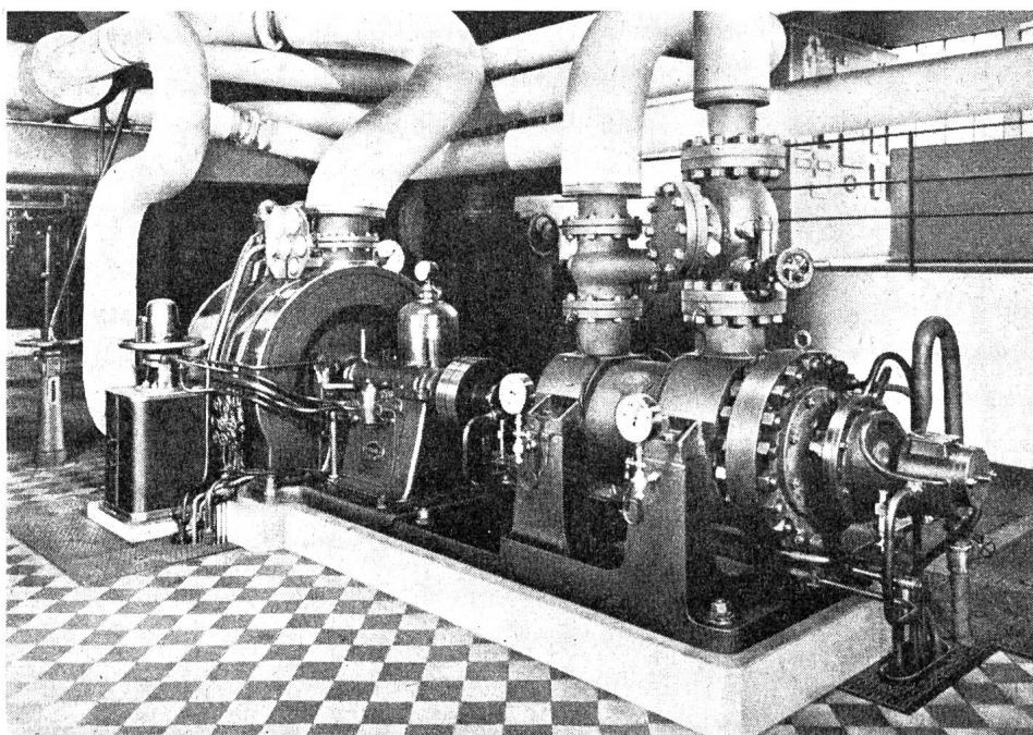
Durch eine Sulzer-Dampfturbine angetriebene siebenstufige Hochdruck-Kessel-Speisepumpe im Dampfkraftwerk Comines der Energie Electrique du Nord de la France; Fördermenge 38,8 l/s, Förderhöhe 657 m.
