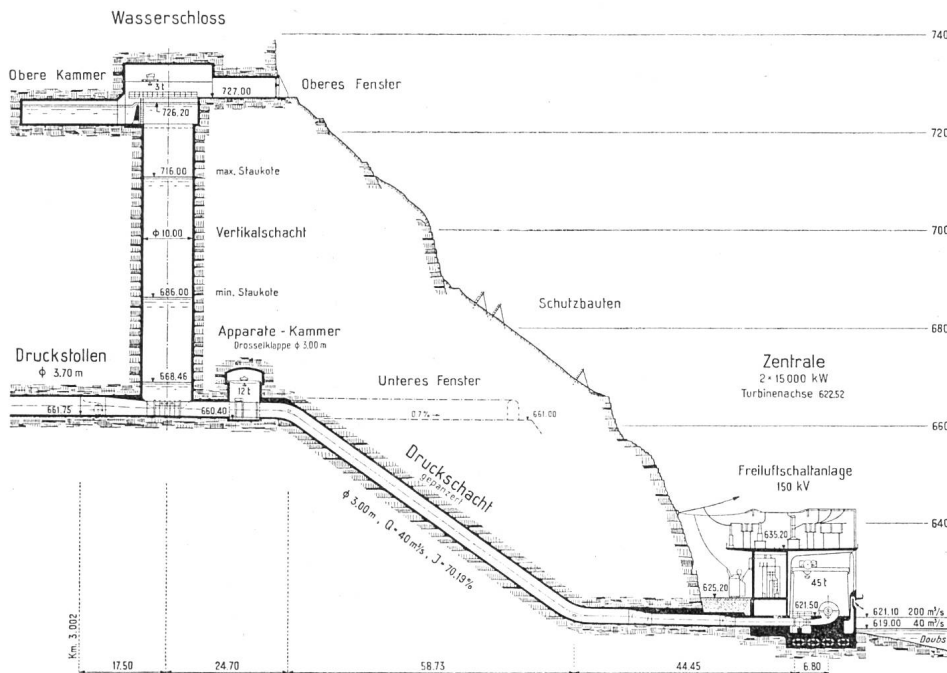
Abb. 12 Wasserschloß, Druckschacht und Zentrale Längsprofil 1 : 1600
