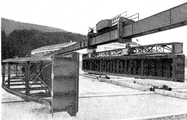
Dammbalken-Versetzkran in Kraftwerk
