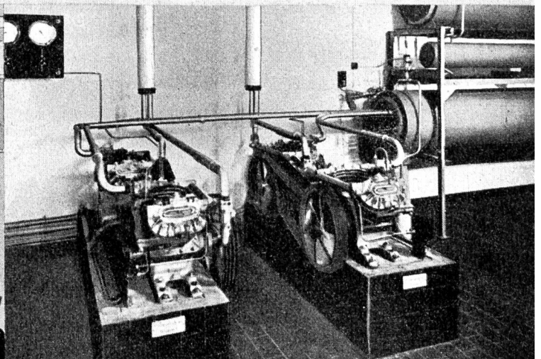
Wärmepumpenanlage im Wohlfahrts- haus der Therma A.-G., Schwanden Gl.
