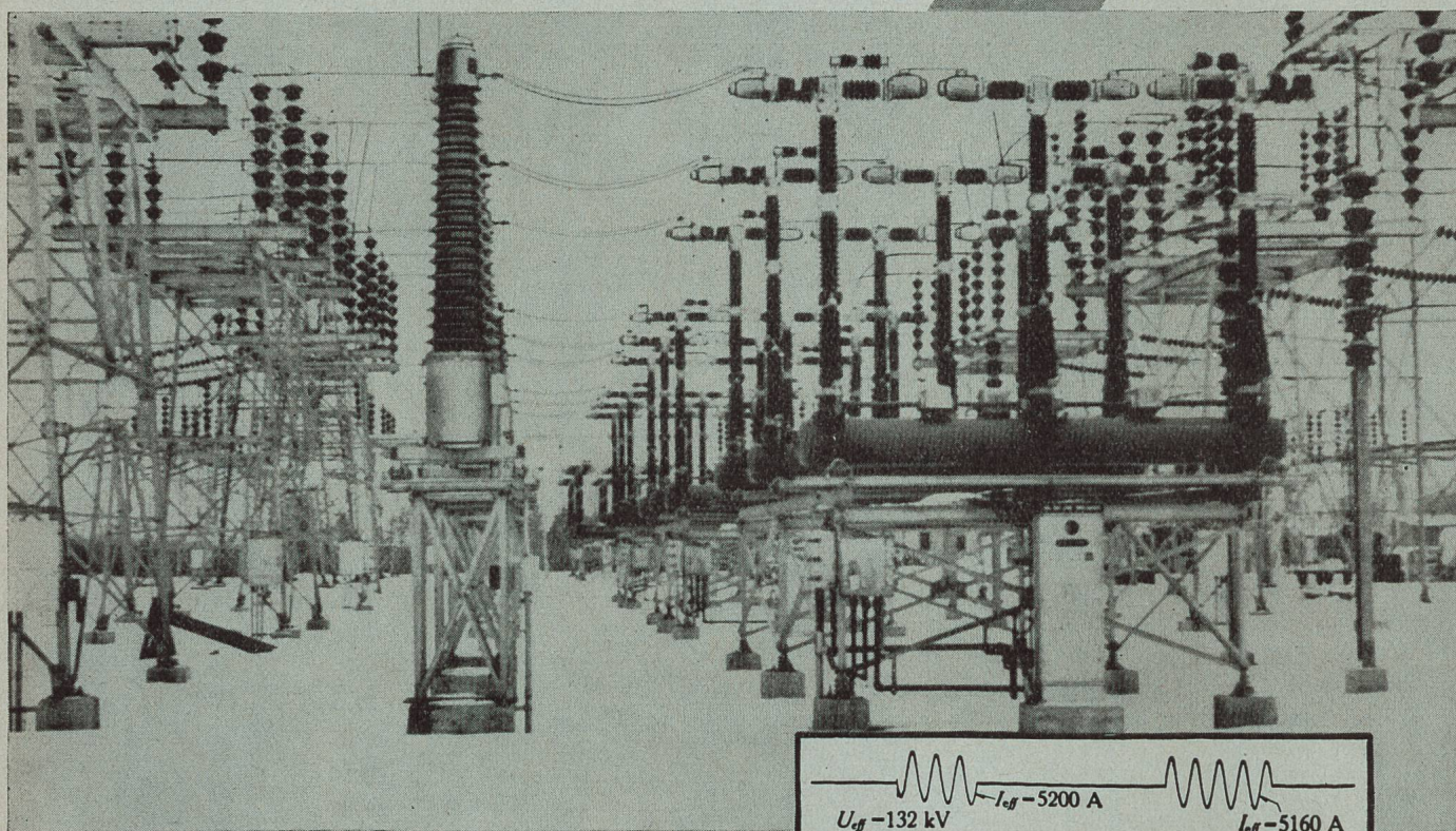
220-kV-Brown Boveri Druckluftschneisschalter in einer kanadischen Freiluftstation
