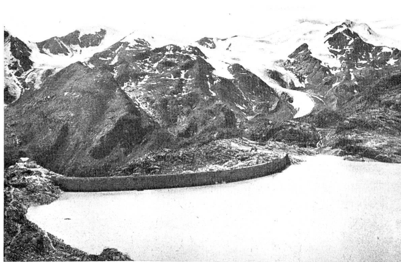
Abb. 13 Stausee Careser in der Ortlergruppe, 2600 m ü. M., der höchstgelegene Speichersee der Ostalpen, Blick gegen Westen mit Vedretta della Mare, rechts M. Cevedale (3774 m) und Zufallspitze (Photo Chiolini-Turconi & Co., Pavia)
