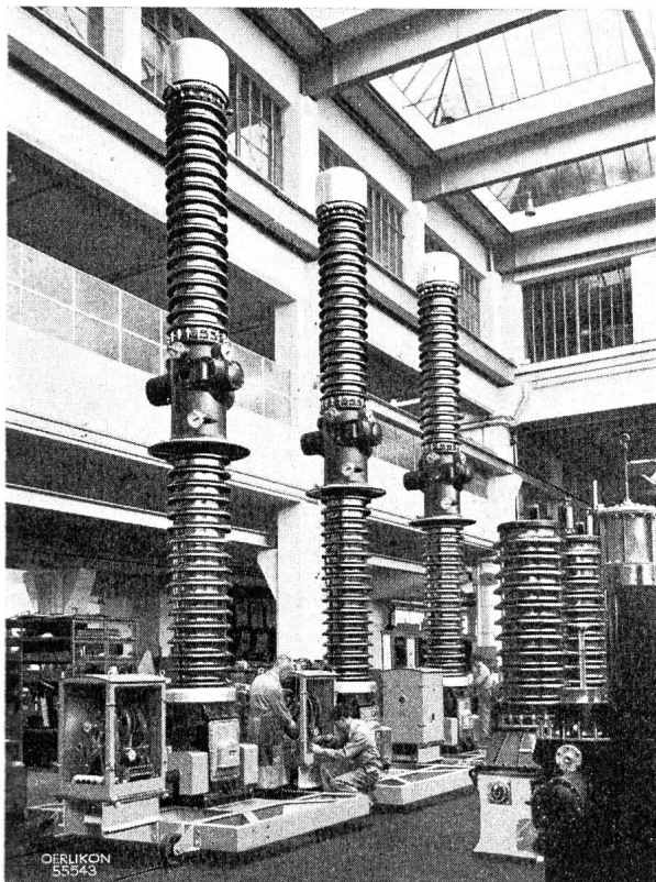
Ölarme Schalter 220 kV in der Montagehalle
