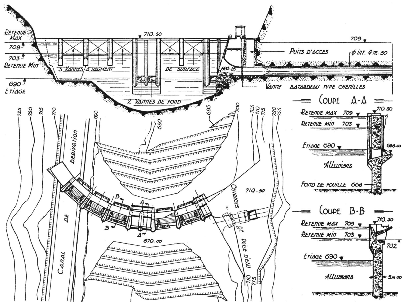
Fig. 12 Barrage et prise d'eau d'Air Ouarda
