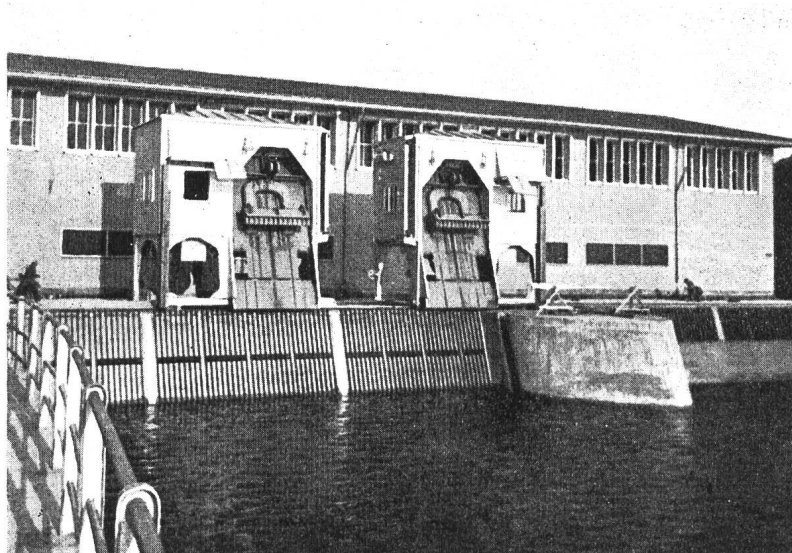
Rechenreinigungsmaschinen
