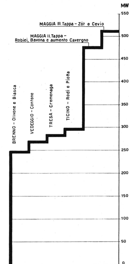
Abb. 12 Installierte Leistung der projektierten tessinischen Kraftwerke
