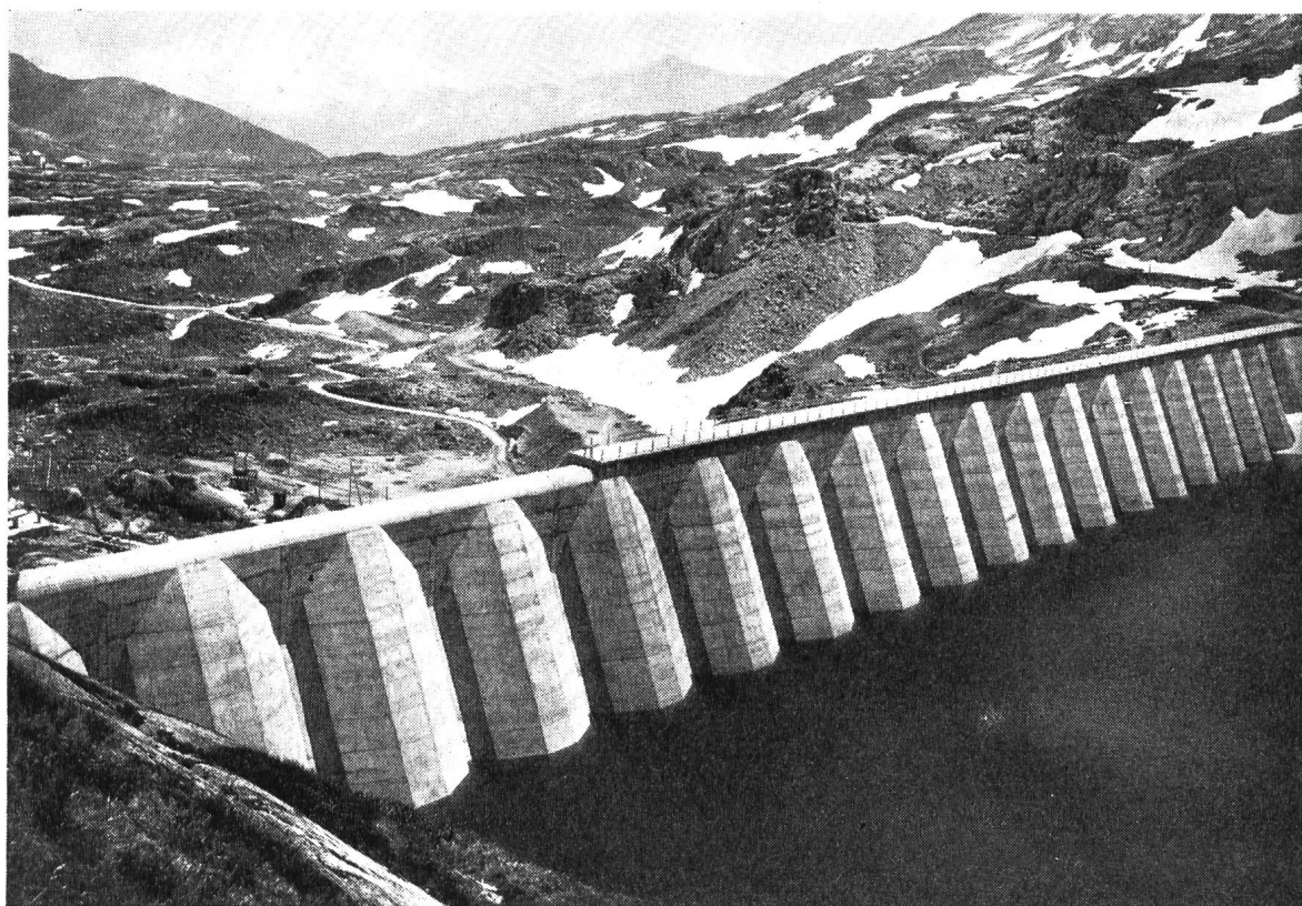
Abb. 5 Staumauer Lucendro, von der Wasserseite gegen die Gotthardpaßhöhe gesehen
