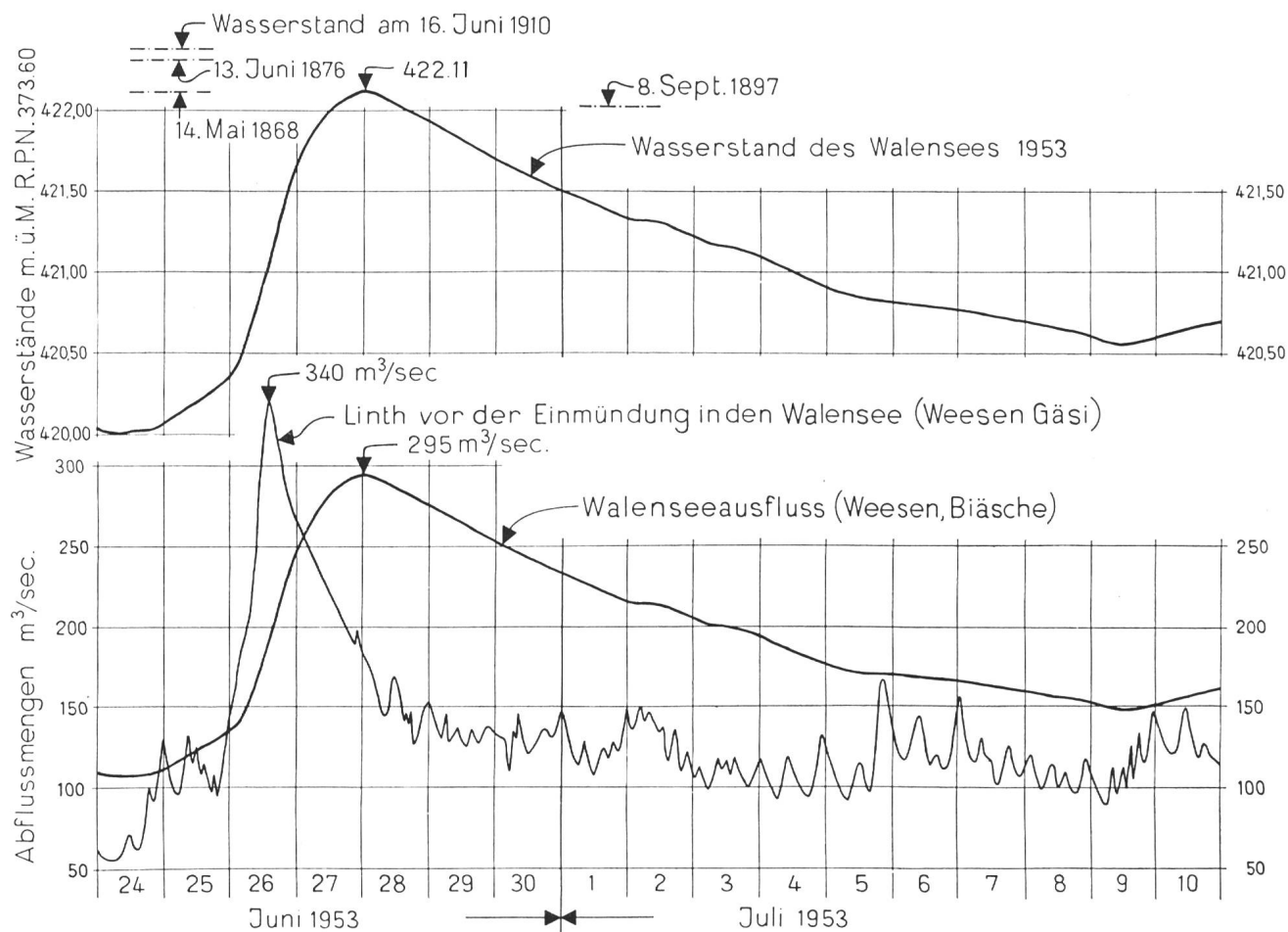
Abb. 3 Ganglinien des Walenseestandes, der Abflußmenge der Linth vor dem Walensee und der Ausflußmenge aus dem Walensee für die Zeit vom 24. 6. bis zum 10. 7. 1953
