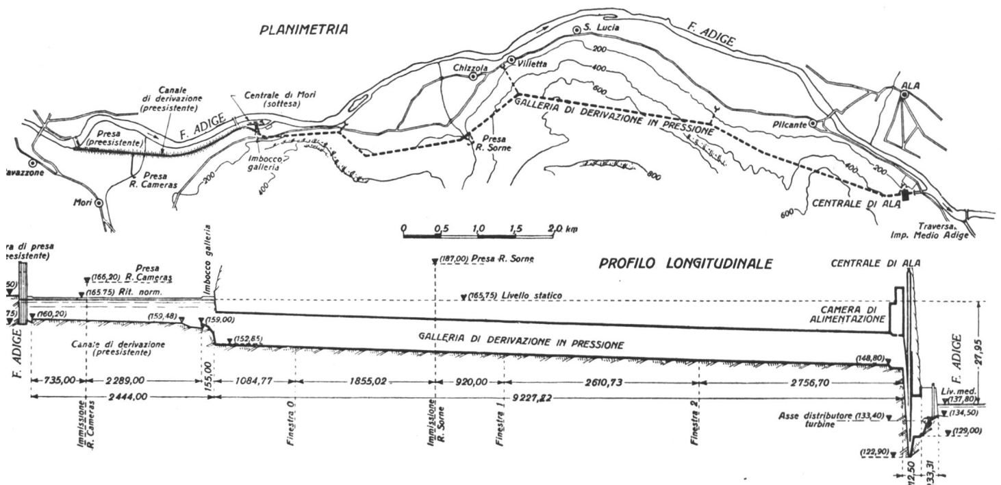
Abb. 35 Kraftwerk Ala an der Etsch, Lageplan und Längsschnitt (aus «Energia Elettrica» 1953, S. 763)
