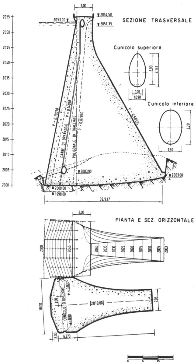
Abb. 25 Pfeiler-Staumauer Fedaia, Querschnitt und Horizontalschnitt 1 : 800
