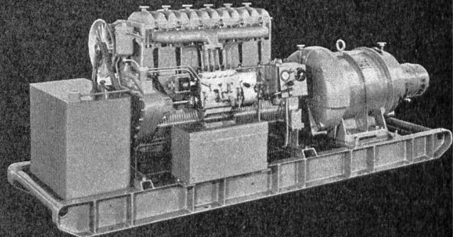
50 kW Notstromgruppe
