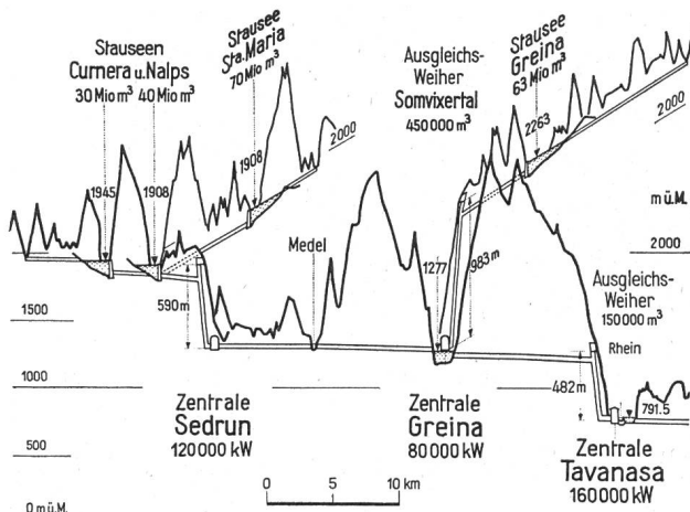
Abb. 3 Schematisches Längenprofil der Vorderrheinkraftwerke, oberer Teil
