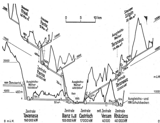
Abb. 4 Schematisches Längenprofil der Vorderrheinkraftwerke, unterer Teil
