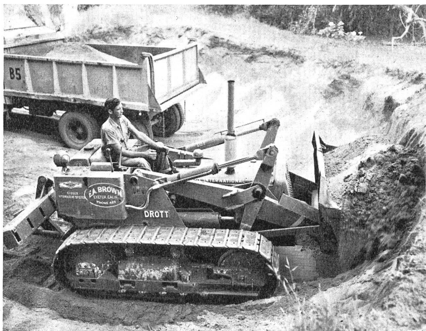
Raupenladeschaufel — International Drott TD-14 A, 1500 l Kübelinhalt, Motor 76 PS
