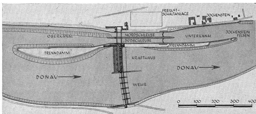
Abb. 18 Jochenstein, Lageplan
