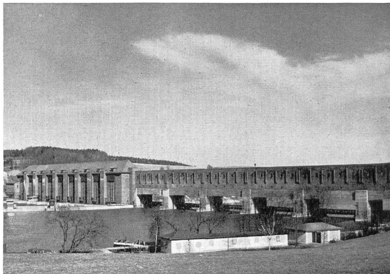
Abb. 17 Kachlerwerk bei Passau (Photo R. Gutscher, Donaukraftwerk Jochenstein AG, Passau)
