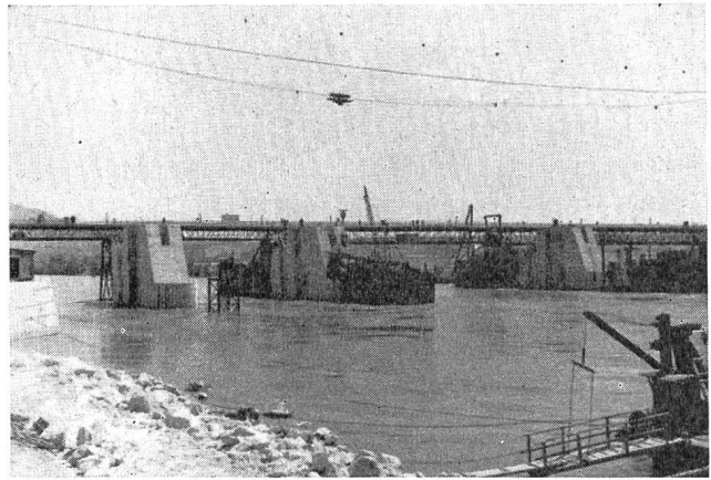
Abb. 2 Kraftwerk Montélimar, Stauwehr bei Rochemaure
