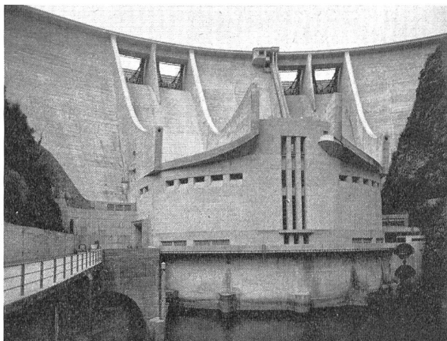
Fig. 6 Barrage de l'Aigle (Energie Electrique de la Moyenne Dordogne: M. Mary). Entreprise L. Ballot; architectes MM. Brachet et Chabbert (Photo H. Baranger)
