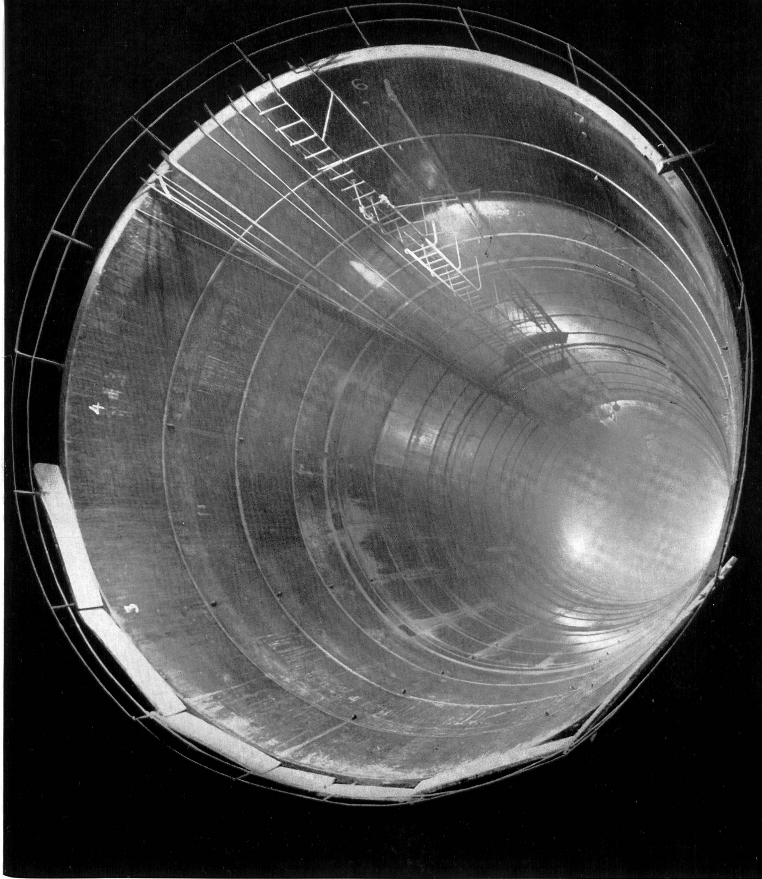
Wasserschloß-Vertikalschacht
