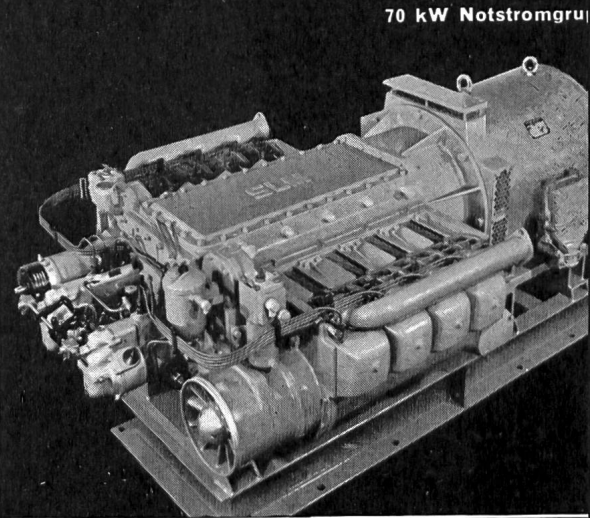
70 kW Notstromgruppe
