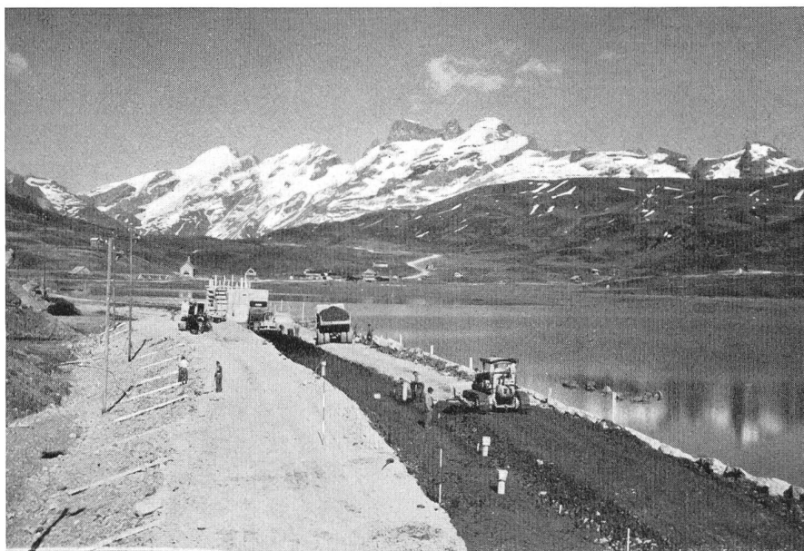
Ausführung der Erddämme Melchsee und Tannensee
