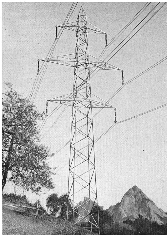
Tragmast der 380 kV-Amsteg-Mettlen-Leitung, ausgerüstet mit Bündelleitern
