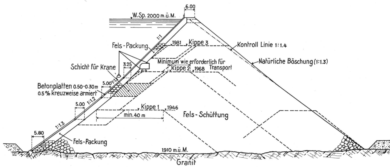
Querschnitt durch einen Felsschütt-Damm mit wasserseitiger Dichtung
