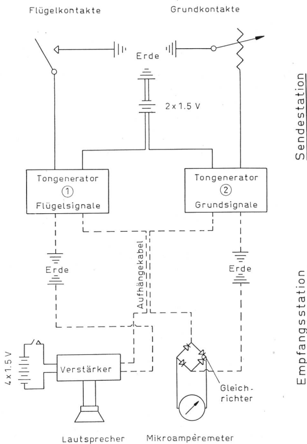
Bild 7 Schema der elektrischen Signalübertragung
