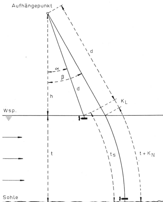
Bild 9 Die Abtrift. Totale Tiefenkorrektur K = K_L + K_N
