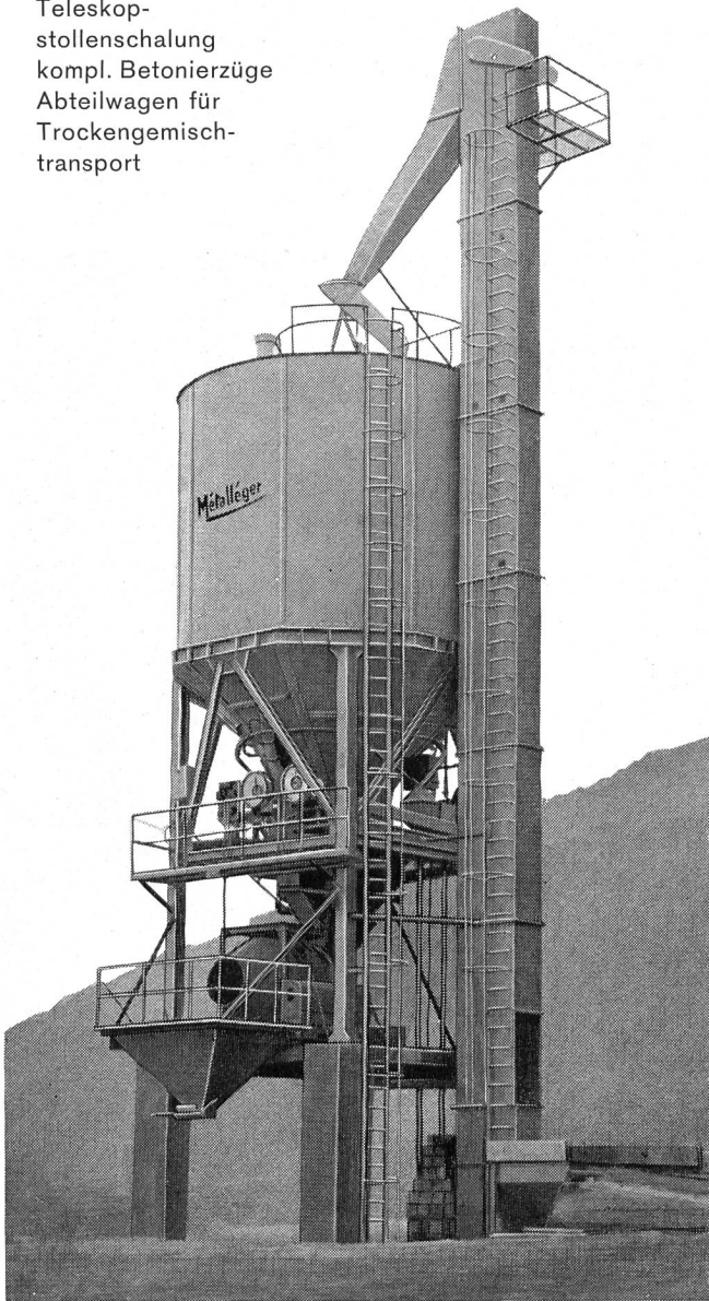
Betondosieranlage Métalléger Typ 130/40 in den Misoxer Kraftwerken
