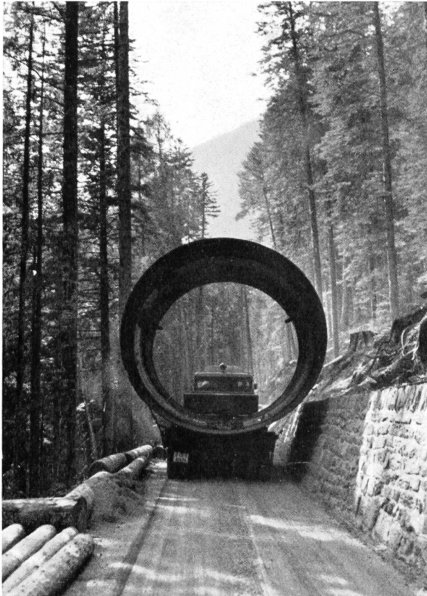
Bild 10 Transport eines Druckrohrs auf einem engen, steilen Waldsträßchen, für die Schachtpanzerung der Stufe Bärenburg-Sils der Kraftwerke Hinterrhein
