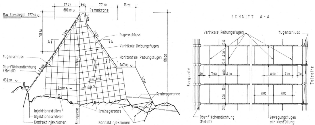
Bild 11 Platani-Damm, Sizilien. Vertikal- und Horizontalschnitte eines aus Betonblöcken aufgebauten Rockfill-Dammes.
