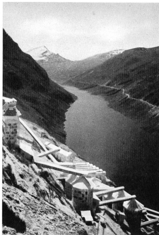
Der vom Pizzo Stella beherrschte Stausee Valle di Lei; erster Teilstau mit rund 32 Mio m 3 (Vollstau 200 Mio m 3 , wovon 197 Mio m 3 Nutzwasser)
