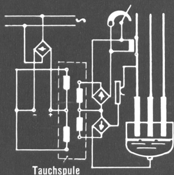
Tauchspule
