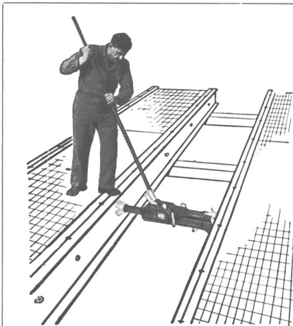
«Simplex» 20-t-Gelenkfußwinde Nr. 2030 mit 480 mm Hub und angepaßtem Ziegenfuß. Das Gas- und Wasserwerk Winterthur hat mit dieser Winde, so wie hier dargestellt, einige tausend Sondierpfähle ausgezogen.
