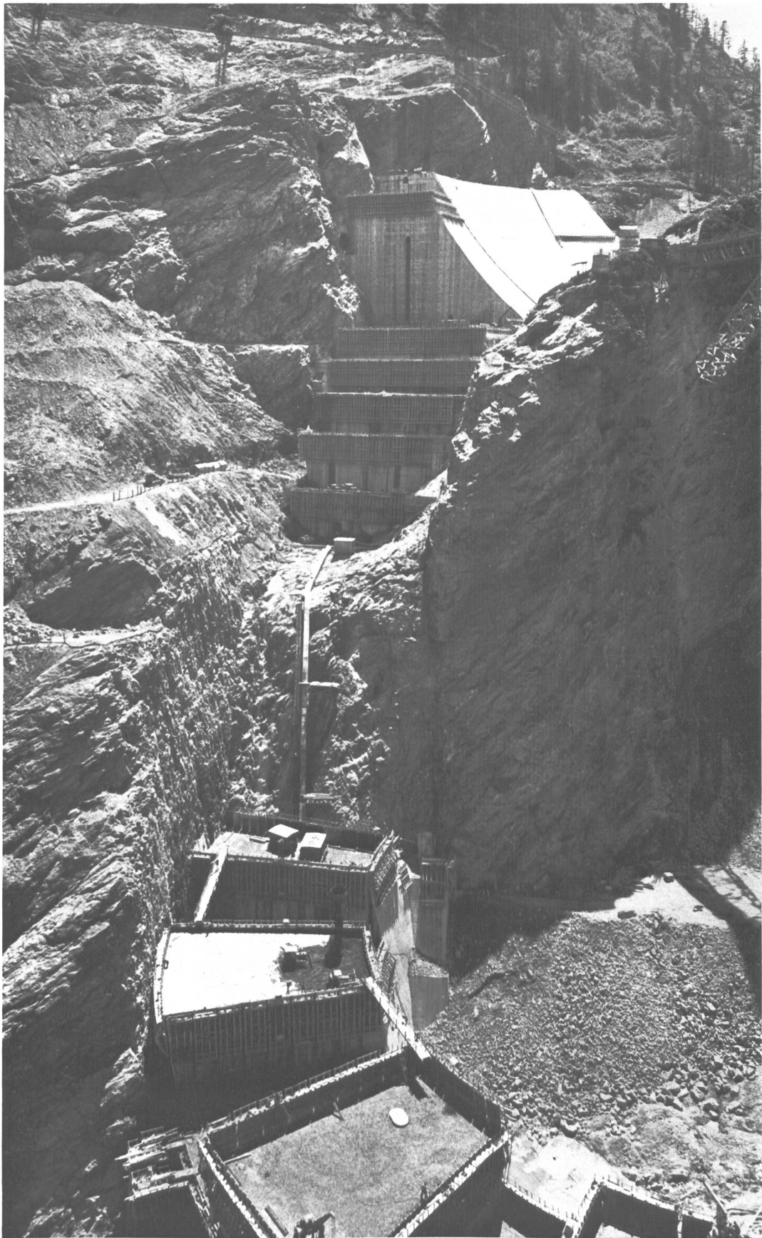
Bild 1 Staumauer Luzzzone der Officine Idroelettriche di Blenio S. A. Bauzustand Ende Juli 1961 mit rund 350 000 m 3 eingebrachtem Beton
