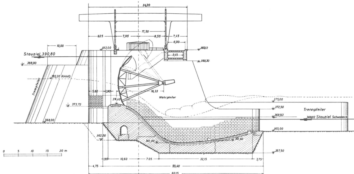
Bild 4 Querschnitt durch das Stauwehr Edling
