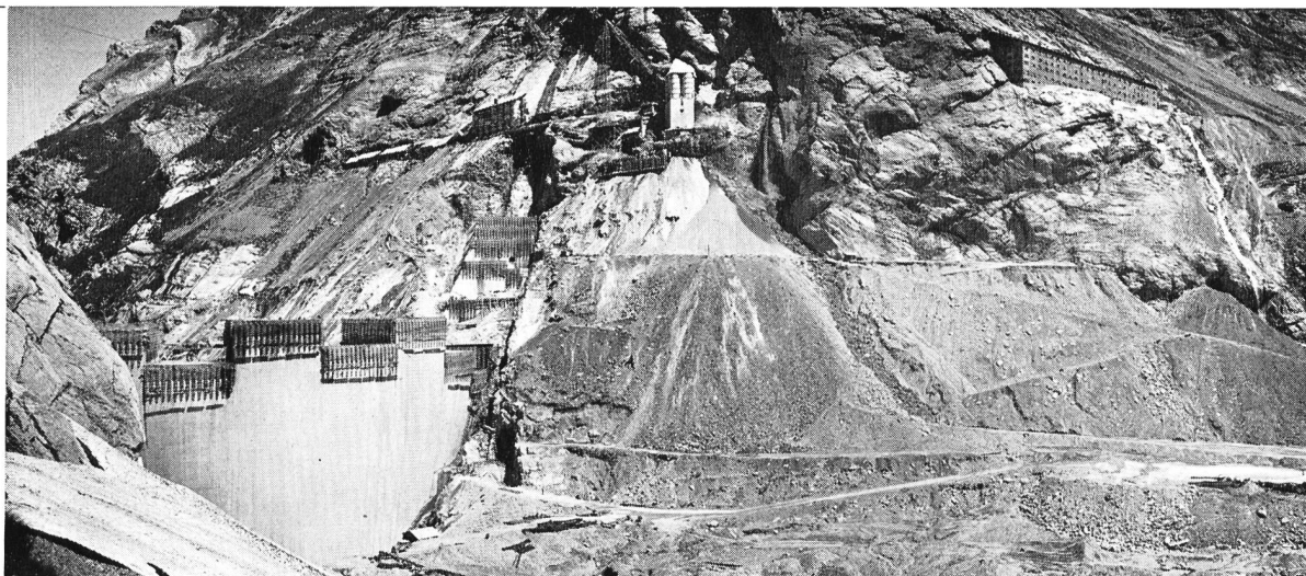
Staumauer Linth-Limmern in Gemeinschaftsarbeit
