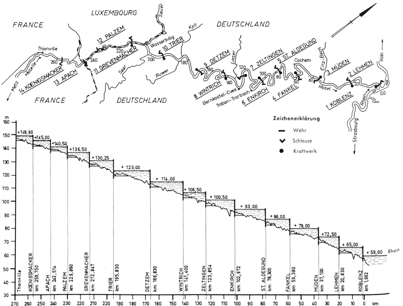
Bild 8 Übersichtsplan, Maßstab 1 : 1 000 000, und Längsschnitt des Ausbauplanes der Mosel zwischen Thionville (Diedenhofen) und Koblenz
