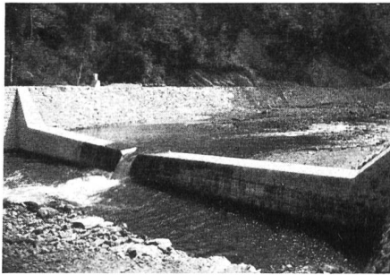
Meßschwelle unterhalb der Staumauer zur Dotierung der Sihl
