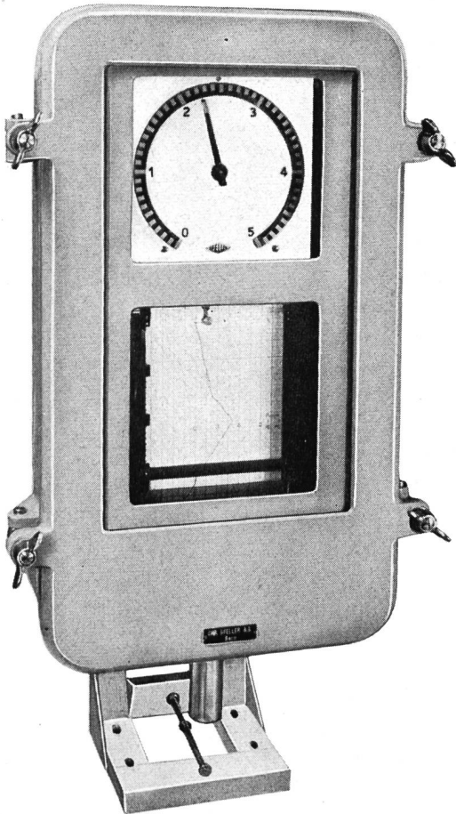
Registrierapparat
