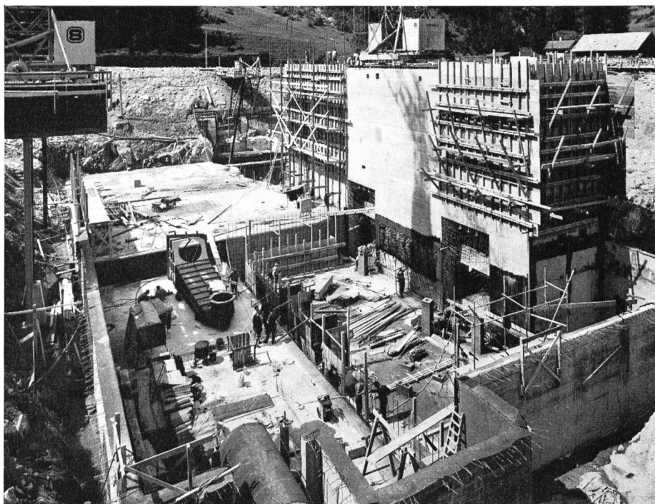
Fig. 16 Baustelle Zentrale Filisur
