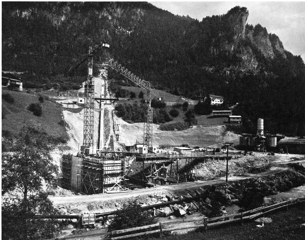
Fig. 15 Uebersicht der Baustelle der Zentrale Filisur und der Druckleitung
