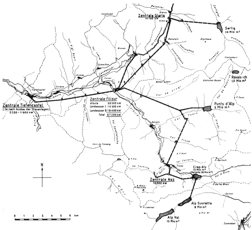
Fig. 2 Lageplan der Wasserkraftnutzung im Albula-Landwasser-Gebiet nach einem Projekt von Ing. Fröté von ca. 1900
