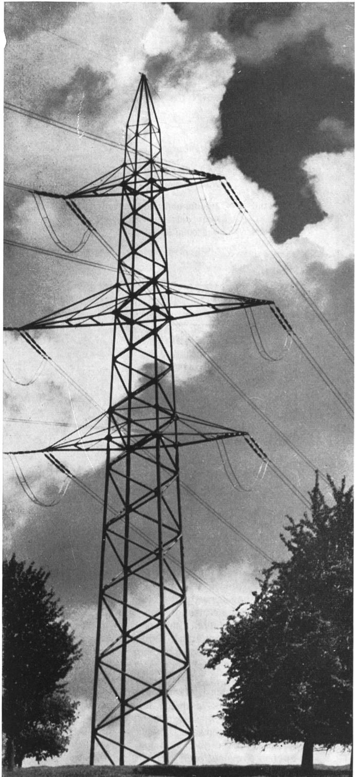
380 kV Abspanneckmast mit Bündelleitern der Leitung Bonaduz-Breite-Laufenburg.
