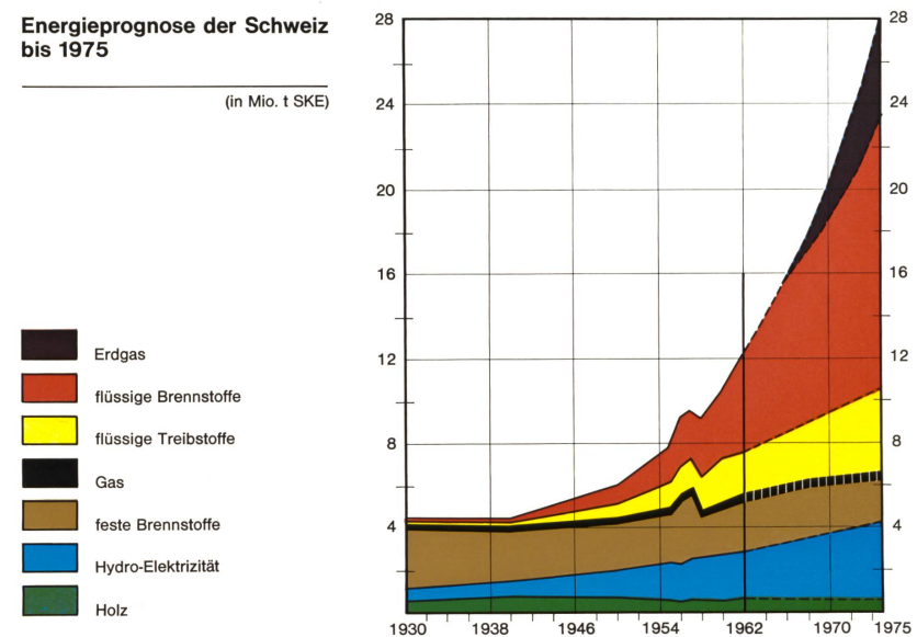
Bild 2 Energieprognose der Schweiz bis 1975
