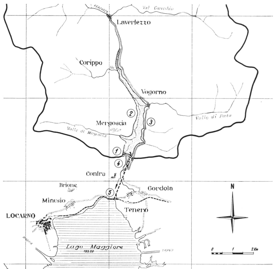
Fig. 2 Plan des installations
