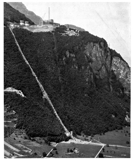
Fig. 3 — Vue aérienne de la centrale de Vouvry, montrant sa position surélevée à environ 450 m au-dessus du fond de la vallée, choisie pour éviter tout danger de pollution de l'air. Le combustible provenant de la raffinerie voisine y est chauffé à 120°C pour être pompé, ainsi que l'eau d'appoint, de la vallée à la centrale.
