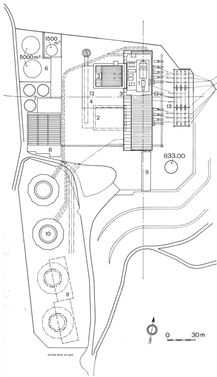
Fig. 2 — La centrale de Vouvry, première grande installation thermique suisse, est équipée de deux groupes turbo-alternateurs identiques d'une puissance unitaire de 150 MW, montés en bloc avec leur chaudière respective. Le combustible lourd est stocké dans deux réservoirs de 5000 m 3 . Comme l'eau de refroidissement n'est pas disponible sur place en quantité suffisante, la température de l'eau est refroidie de 22 à 14 °C, en circuit fermé, dans deux tours de réfrigération par groupe. L'eau évaporée est remplacée par pompage du canal Stockalper.
