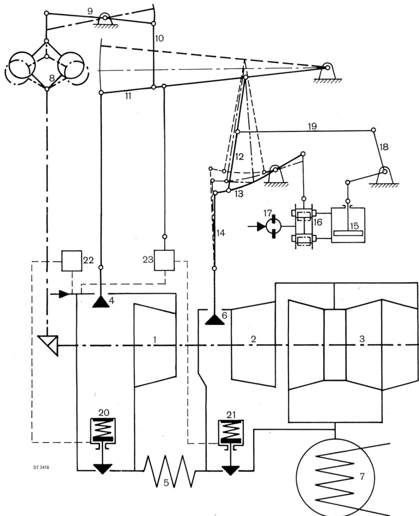
Fig. 12 La régulation compound, développée par Escher Wyss, interrompt non seulement, en cas de décharge, l'arrivée de vapeur vive dans le corps haute pression, mais aussi, par les soupapes d'interception, celle dans le corps moyenne pression. La fermeture simultanée et rapide de ces deux soupapes par le pendule accélérométrique maintient, même en cas de délestage total, la vitesse en dessous des valeurs de déclenchement des dispositifs de sécurité.
