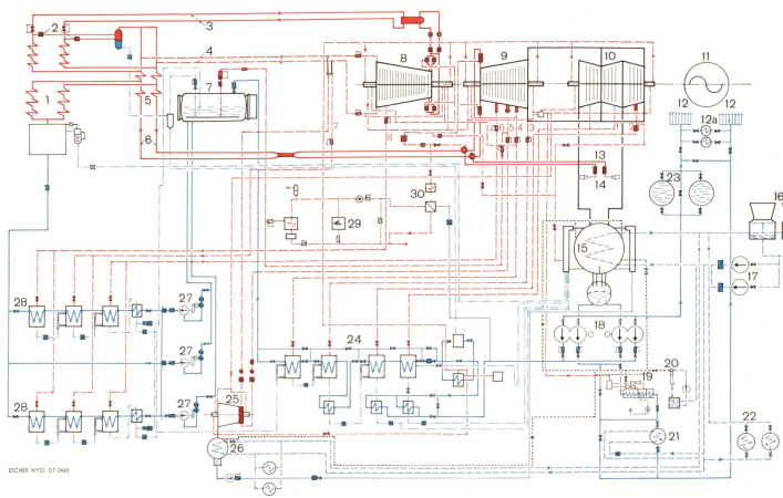
Fig. 7 — Schéma des conduites pour la vapeur vive de 190 kg/cm 2 à 540 °C, le soutirage, l'eau de refroidissement, le condensat, l'eau d'alimentation et l'air.
