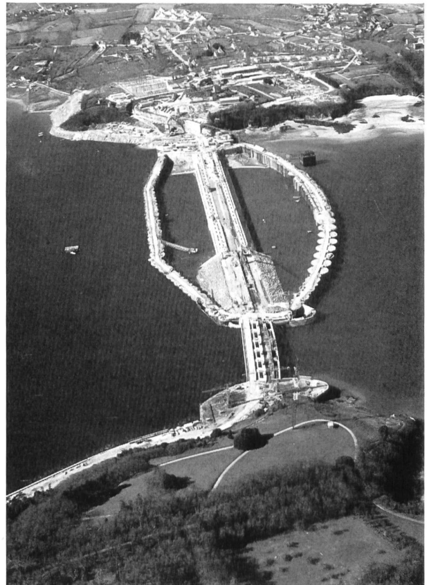
Gesamtübersicht des Gezeitenkraftwerks «La Rance». Im Vordergrund des Bildes das Wehr mit seinen sechs Öffnungen; in der Bildmitte — in der gefluteten Baugrubenumschliessung — der Damm mit dem angebauten Maschinenhaus, in dem auch der Kommandoraum untergebracht ist; im Hintergrund die Schiffsschleuse, Strassenzufahrt und 225 kV Umspannstation.
