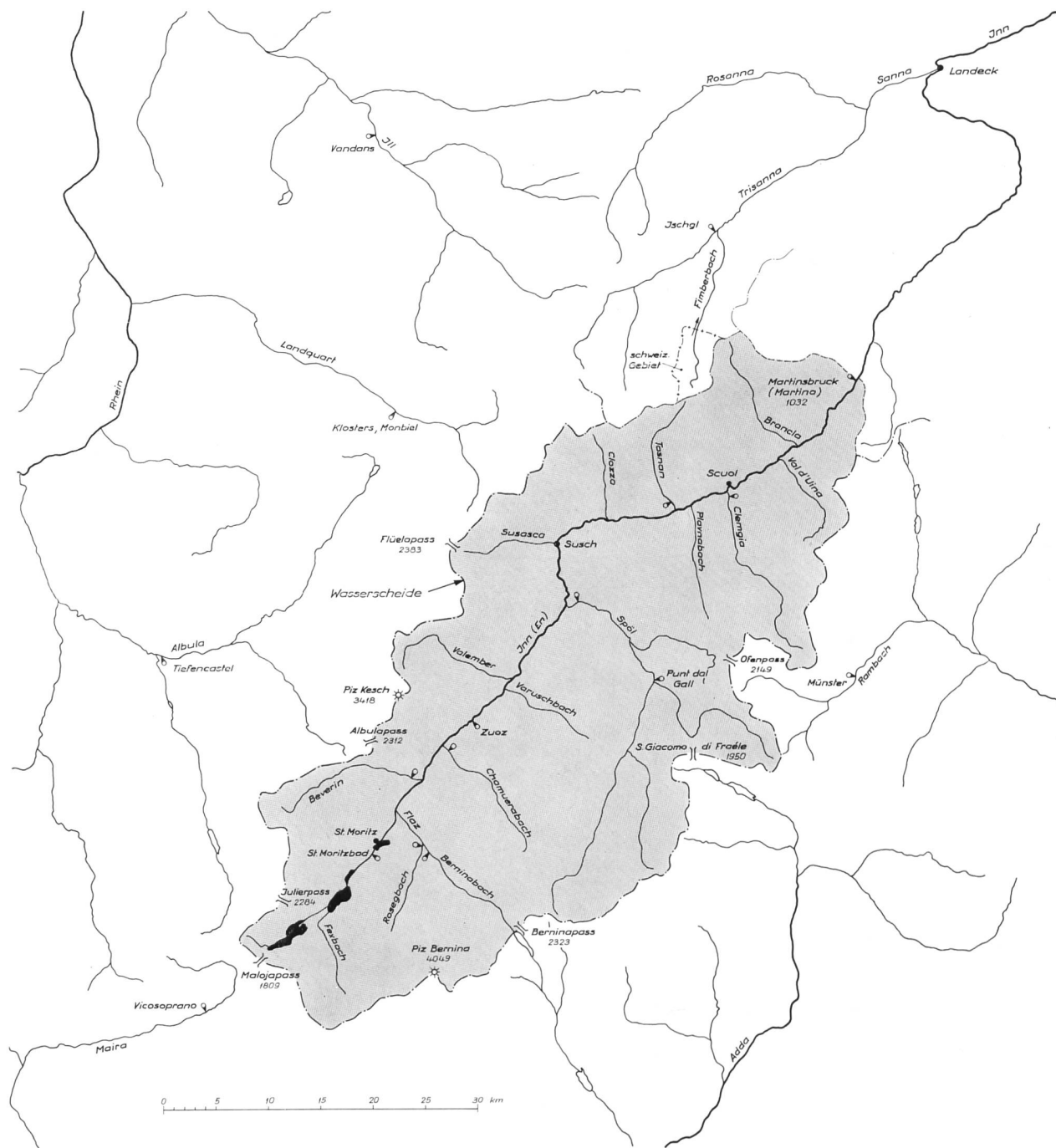
Bild 6 Uebersicht über das Inngebiet oberhalb Martinsbruck/Martina. Hauptwasserscheide, Gewässernetz, Lage der im Text erwähnten Wasserserssstationen.
