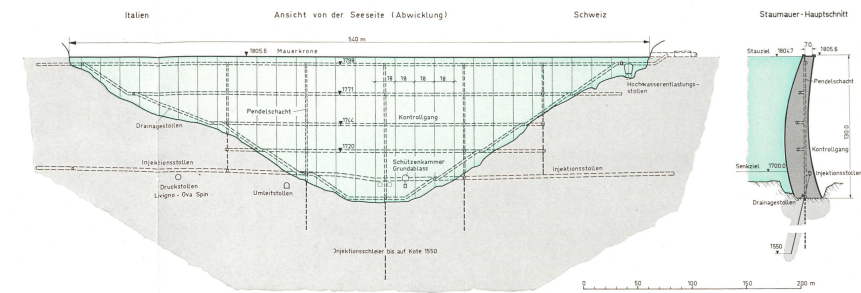
Bild 46 Ansicht von der Seeseite und Staumauerhauptschnitt
