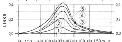
VERFORMUNGEN IN LÄNGSRICHTUNG
