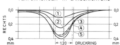
VERFORMUNGEN IN LÄNGSRICHTUNG
