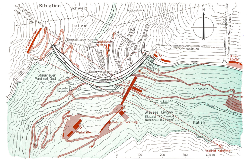
Bild 45 Lageplan
