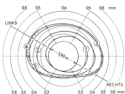
RADIALE VERFORMUNGEN NACH INJEKTION
