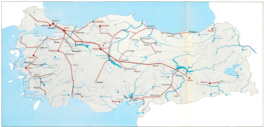
Bild 20 Speicherseen, Kraftwerke und Hochspannungsleitungen in der Türkei (Plan SWV 1967)
