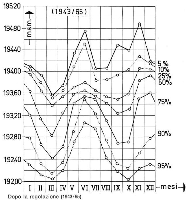
Figura 2 Curve di probabilità dal 5% al 95% per le variazioni medie giornaliere del lago al limnografo di Locarno, per il periodo a regime naturale (1927—1942) e a regime regolato (1943—1965).
