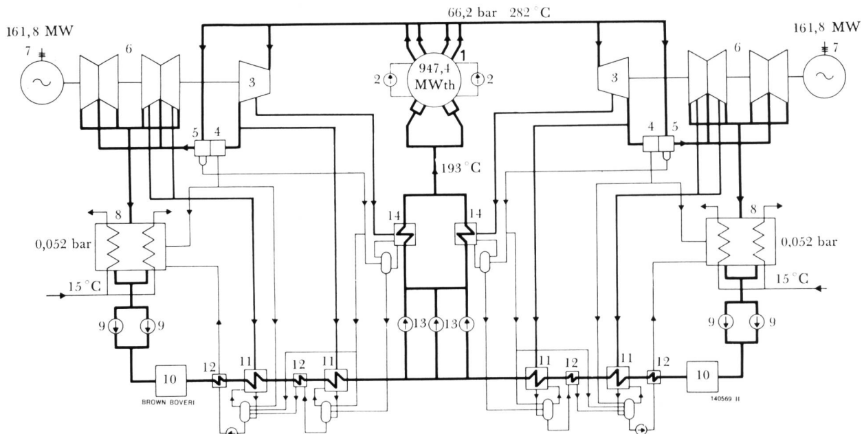
Bild 2 Vereinfachtes Wärmeschaltbild
