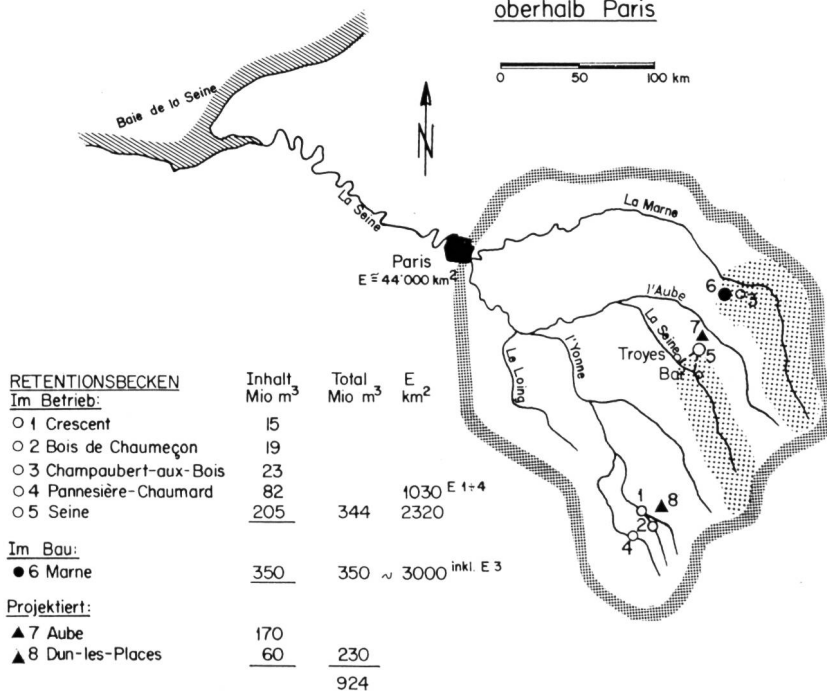
Retentionsbecken im Einzugsgebiet der Seine oberhalb Paris
