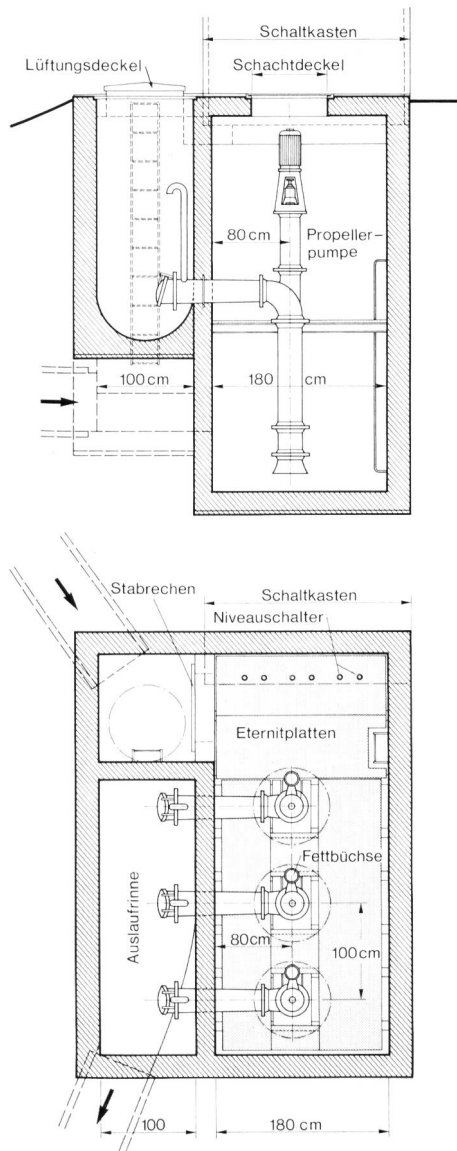
Bild 4 Horizontal- und Vertikalschnitt für den Pumpwerktypus mit Einheiten à 100 l/s Nennleistung.
